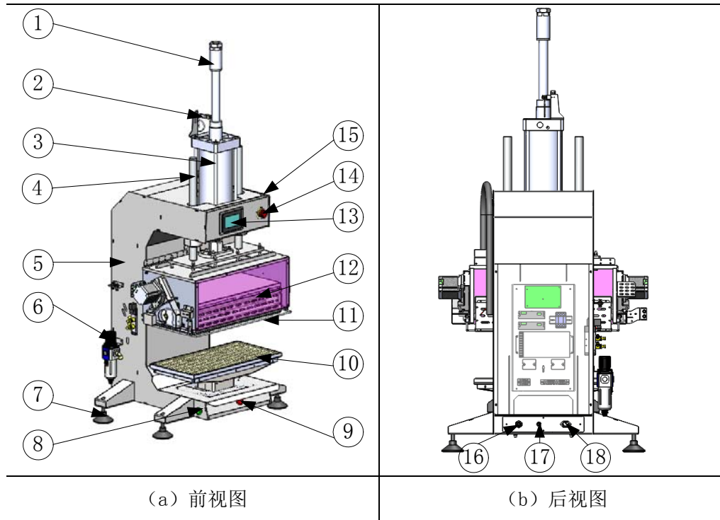
图 2 机器部件名称
