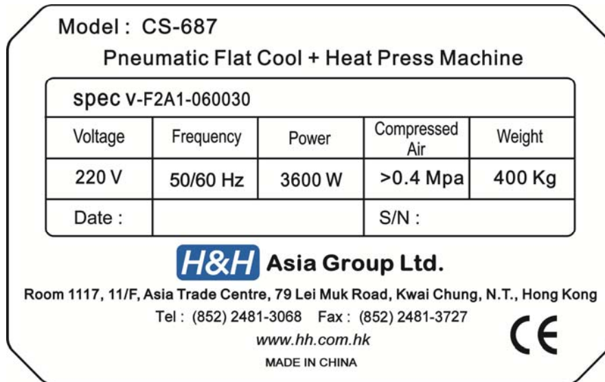
图 1 设备铭牌
